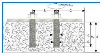
FIGURA 2 - Detalle de instalacion tipica para varilla rosca o barra de construccion.
