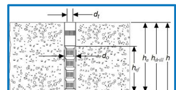
FIGURA 3 - Detalle de instalacion tipica para insertos internamente roscados.
